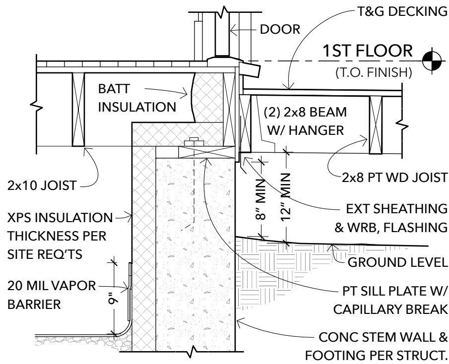
1A FOUNDATION OPT A: CRAWLSPACE SCALE: 1" = 1'-0" CONDITIONED CRAWLSPACE
