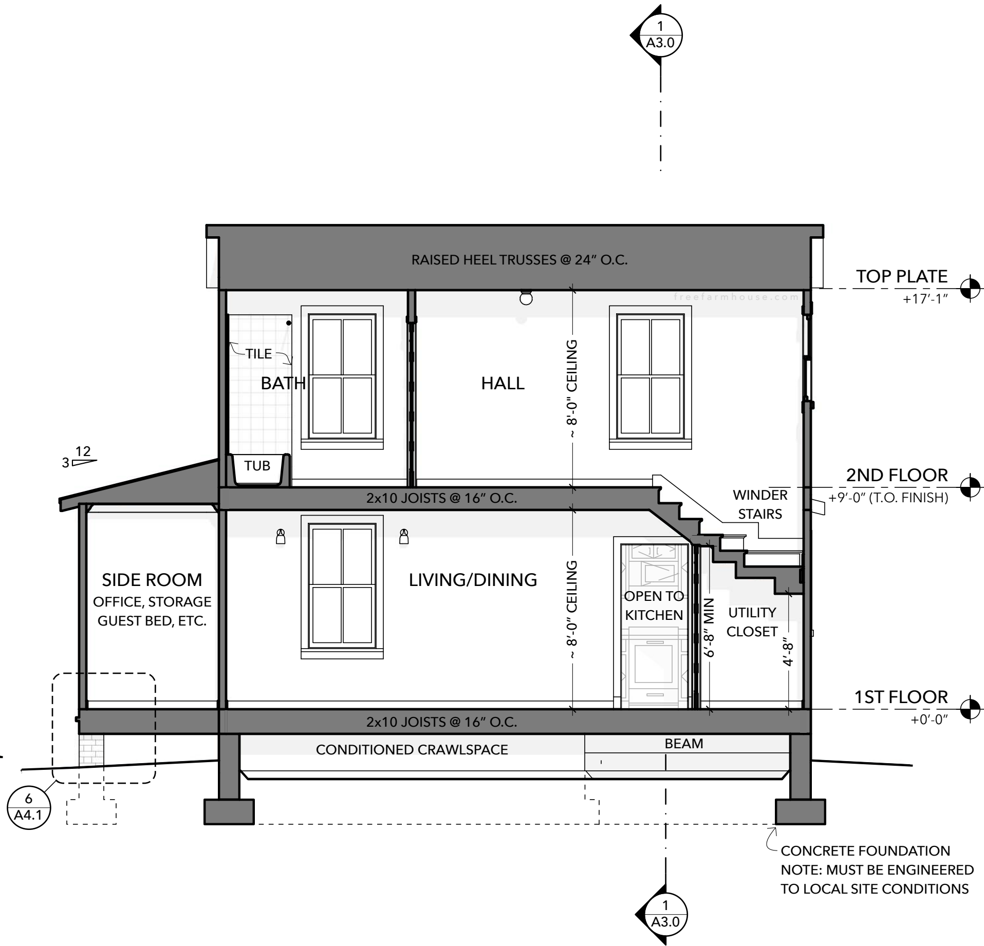
2 LONGITUDINAL SECTION SCALE: 1/4" = 1'-0"
