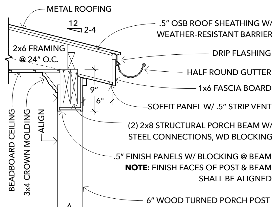
3 PORCH EAVE DETAIL SCALE: 1" = 1'-0"
